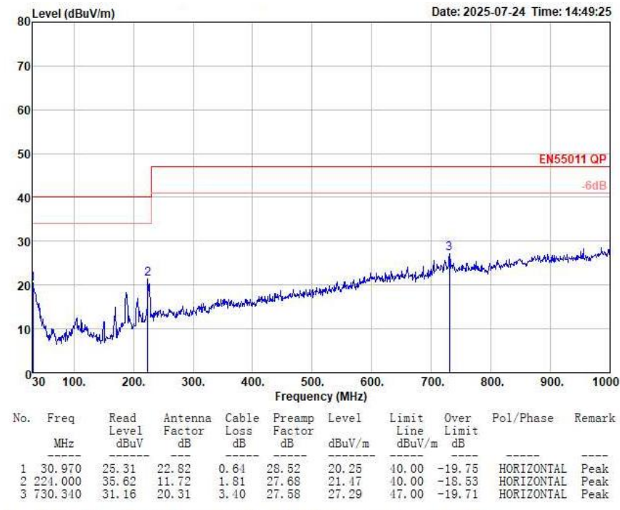
图 6-7 辐射测试水平方向
