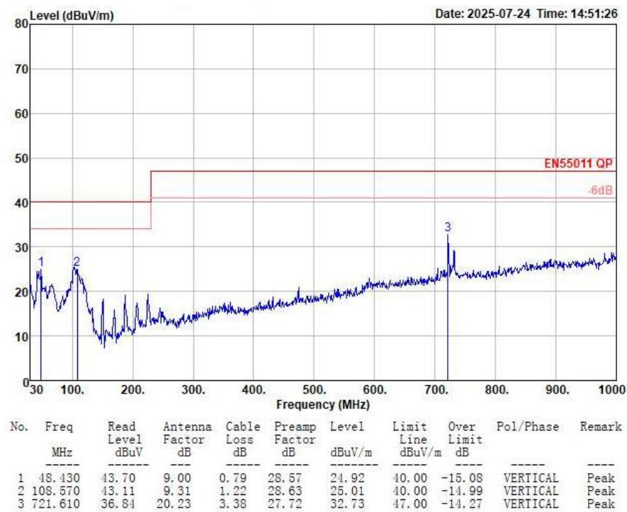
图 6-8 辐射测试垂直方向
