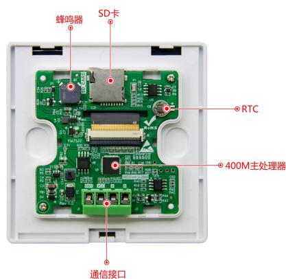
图 1-2 硬件配置图
